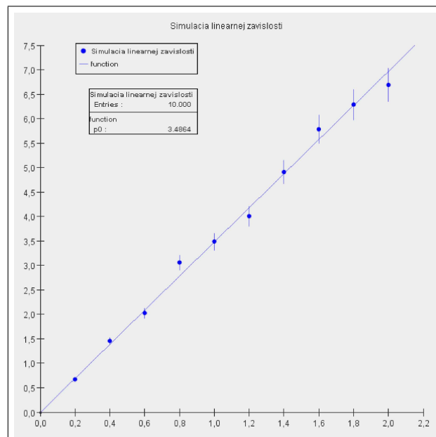
Obrázok 5.14: Example8
