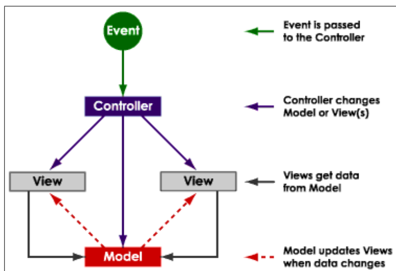
Obrázok 2.2: Model–View–Controller
