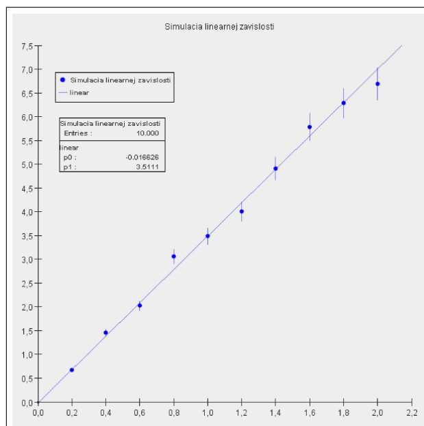
Obrázok 5.13: Example7
