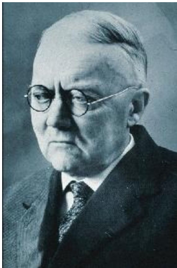
Ernst Öpik 1893 – 1985
